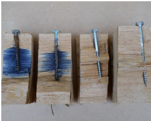
Stahlschrauben unterschiedlicher Güte in neuem Eichenbauholz
